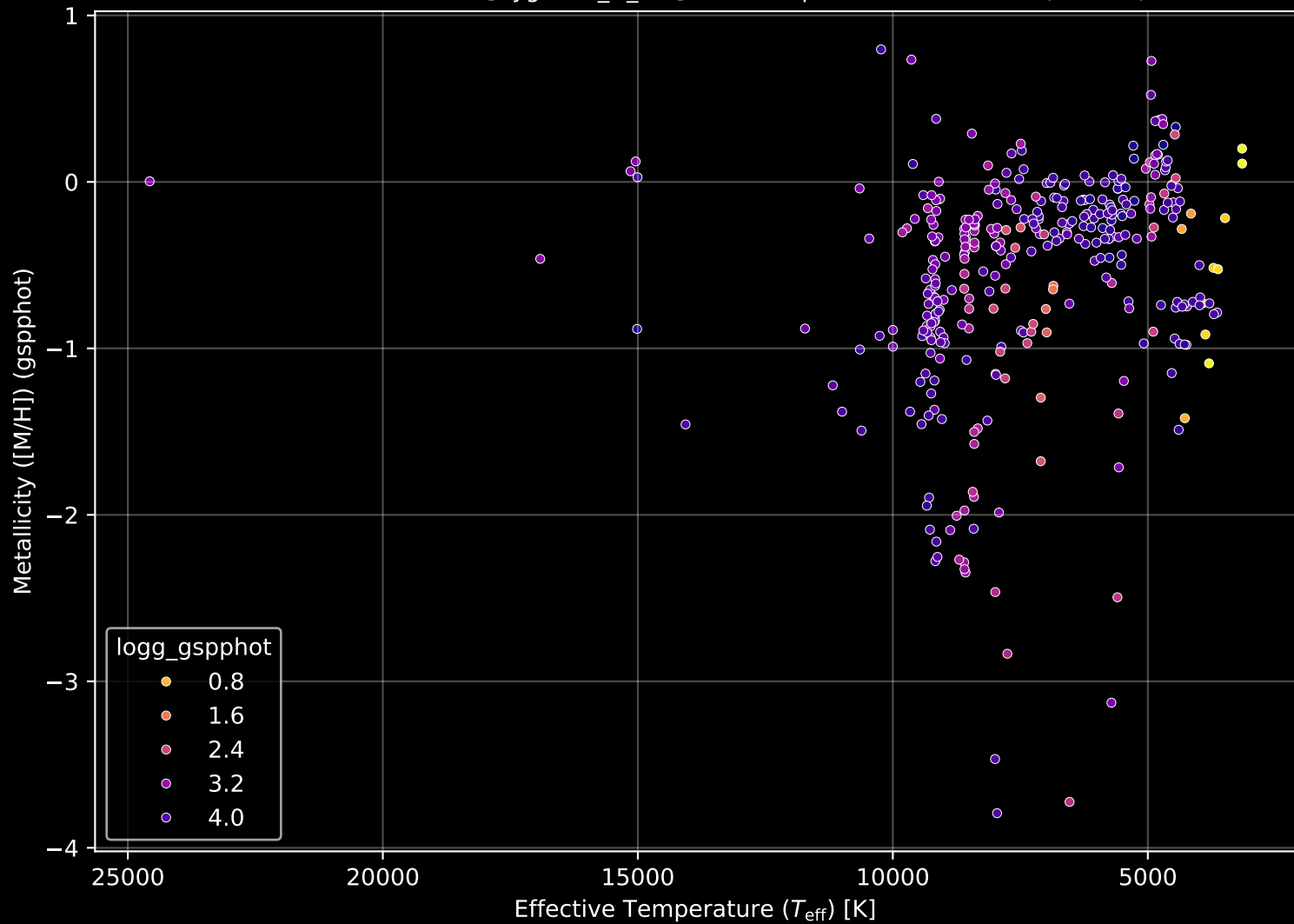
APOGEE DR17 Field: [CygnusX_N_btx] Stellar Population Parameters (n= 349)
